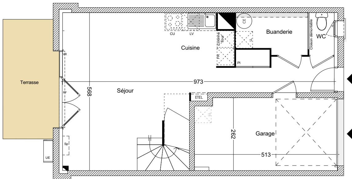
Plan RDC
