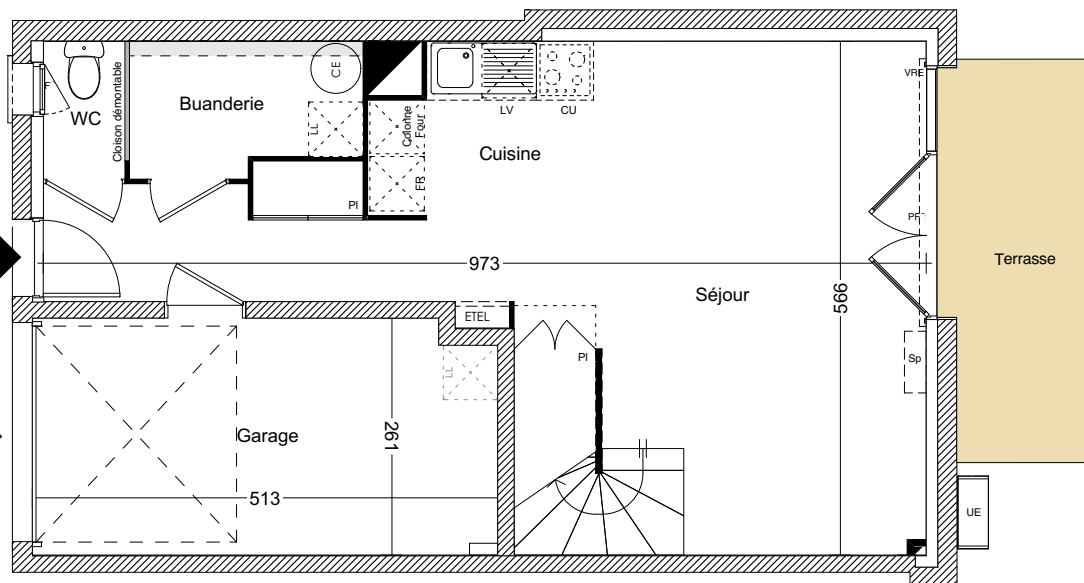
Plan RDC
