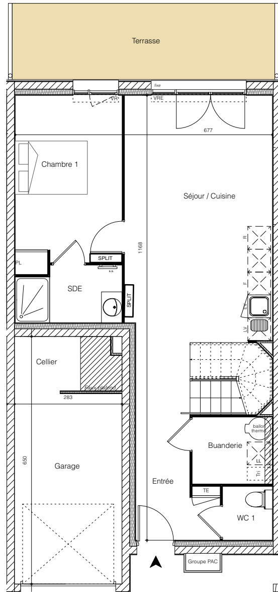
Plan RDC
