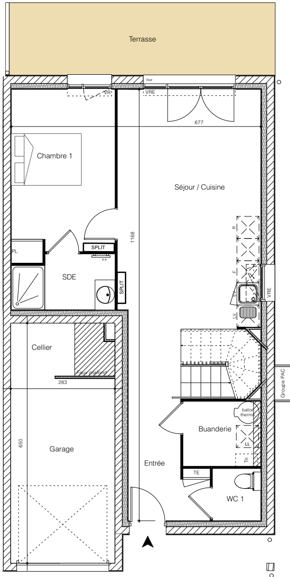
Plan RDC
