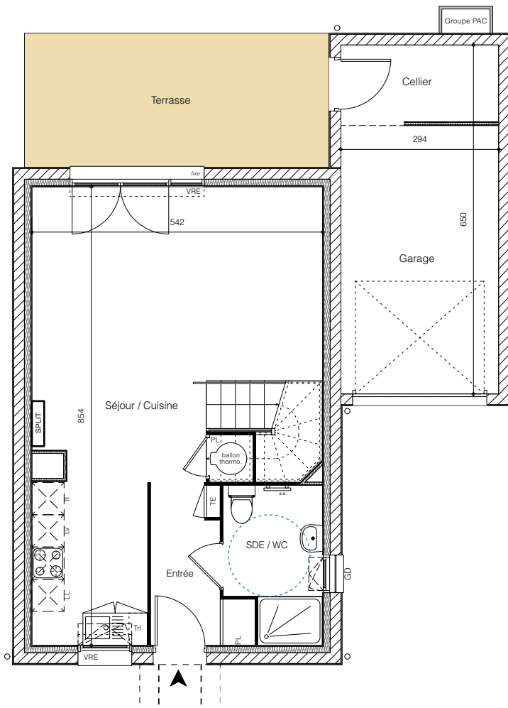
Plan RDC
